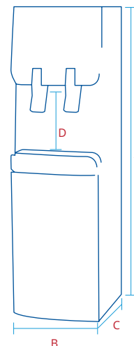
Dimensiones (a x b x c x d en mm): 1025 x 300 x 340 x 175
