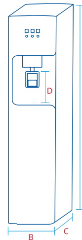
Dimensiones (a x b x c x d en mm): 1100 x 260 x 347 x 160
